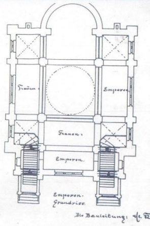
Die Synagoge im Grundriß
